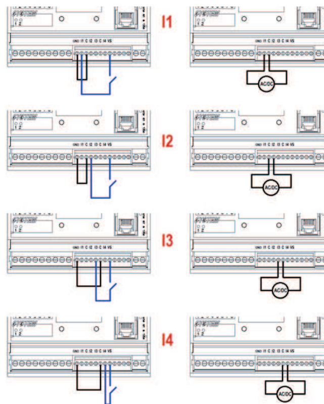
Рисунок 14: Пример соединения входов со станцией I/O
