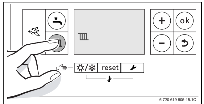
Рис. 4 Дисплей отопления
