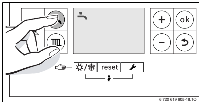
Рис. 8 Дисплей ГВС
