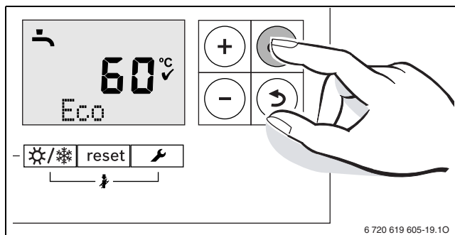
Рис. 9 Параметры экорегима
