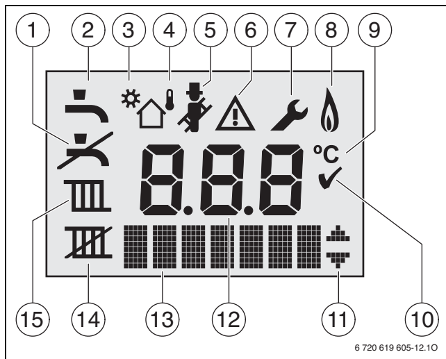
Рис. 2 Отображаемые символы
